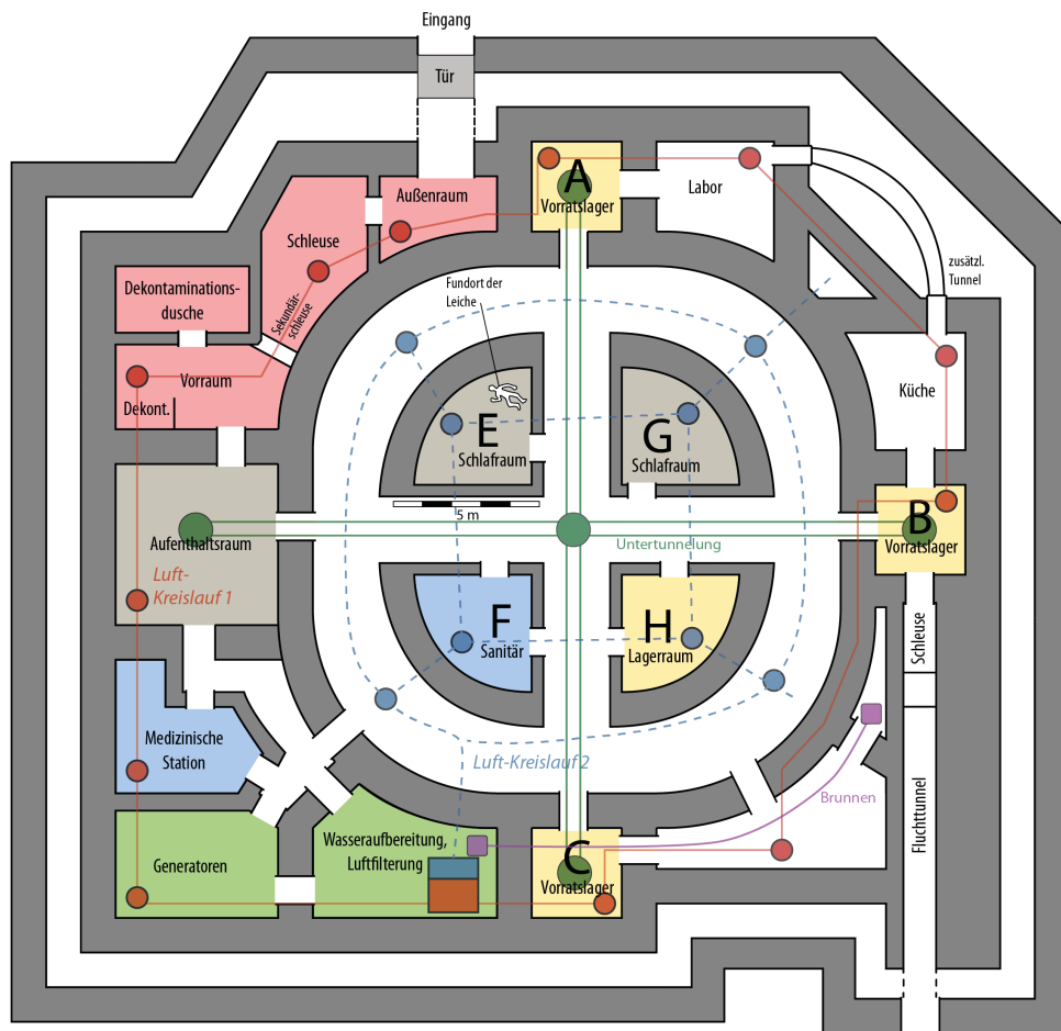
Abbildung 1: Grundriss des Bunkers.
